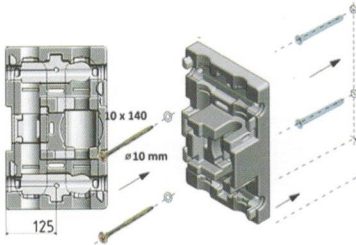
Рис. Настенное крепление насосных групп
