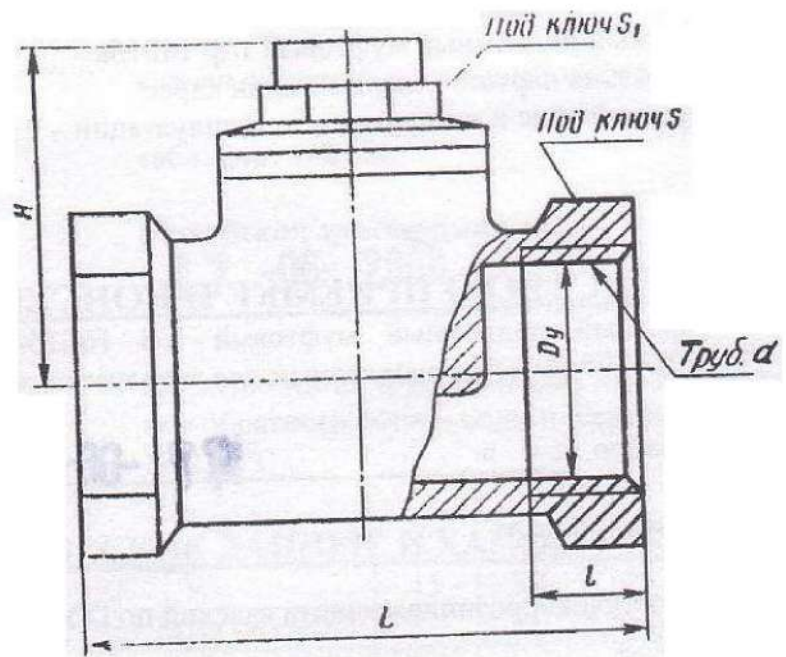
Рис. Клапан обратный подъемный муфтовый 16Б16к
