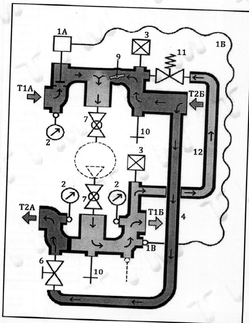
6. Принцип действия насосно-смесительного узла
