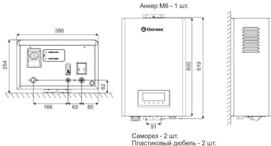
Рис. 6. Монтажные размеры
