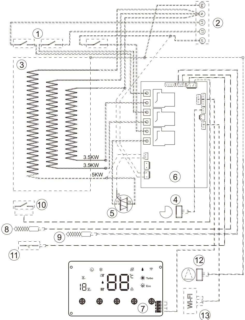
Рис. 15. Электрическая схема THERMEX Grizzly 5-12 Wi-Fi
