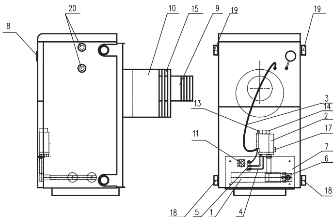
Рисунок 1. Устройство котла с коаксиальным трактом
