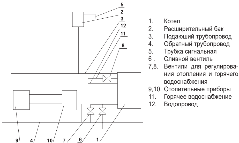
Рисунок 4. Схема подключения котла к отопительной системе с естественной циркуляцией теплоносителя
