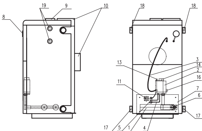
Рисунок 2. Устройство котла с раздельным трактом
