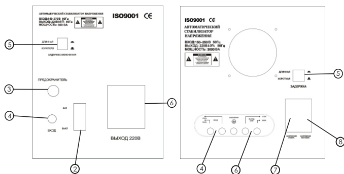
Рис. 2 Вид сзади
