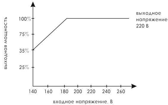
Рис. 3 Нагрузочная характеристика
