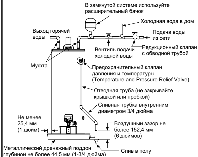
Рисунок 13 Установка водопровода
