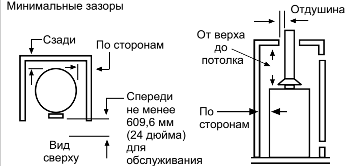
Рисунок 2 Минимальные зазоры
