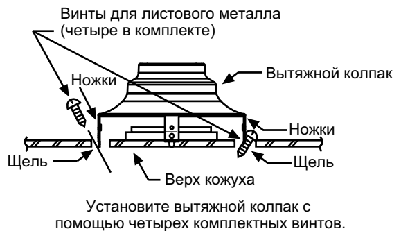
Рисунок 9 Установка вытяжного колпака
